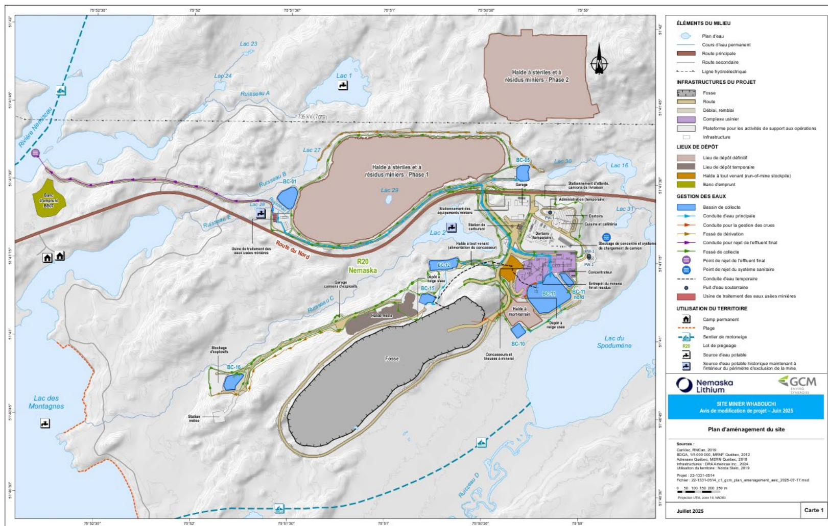
Figure 1. Plan d'aménagement du site du projet
